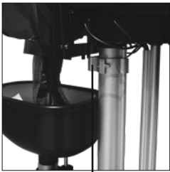
Support frame Vorrichtung, zur Anbringung des Netzes Support de fixation du filet
